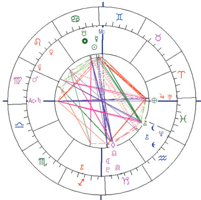
De gedeeltelijke maansverduistering van 26 juni 2010 12:30 MET Greenwich.
